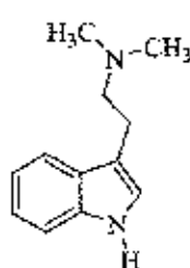
DMT
