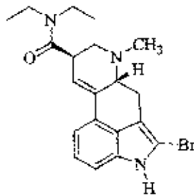
BOL
