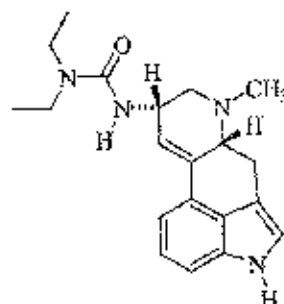
Lisuride
