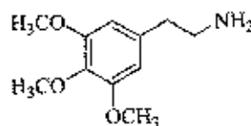
Mescaline
