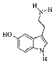
Serotonin; 5-HT
