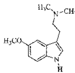
5-Methoxy-DMT
